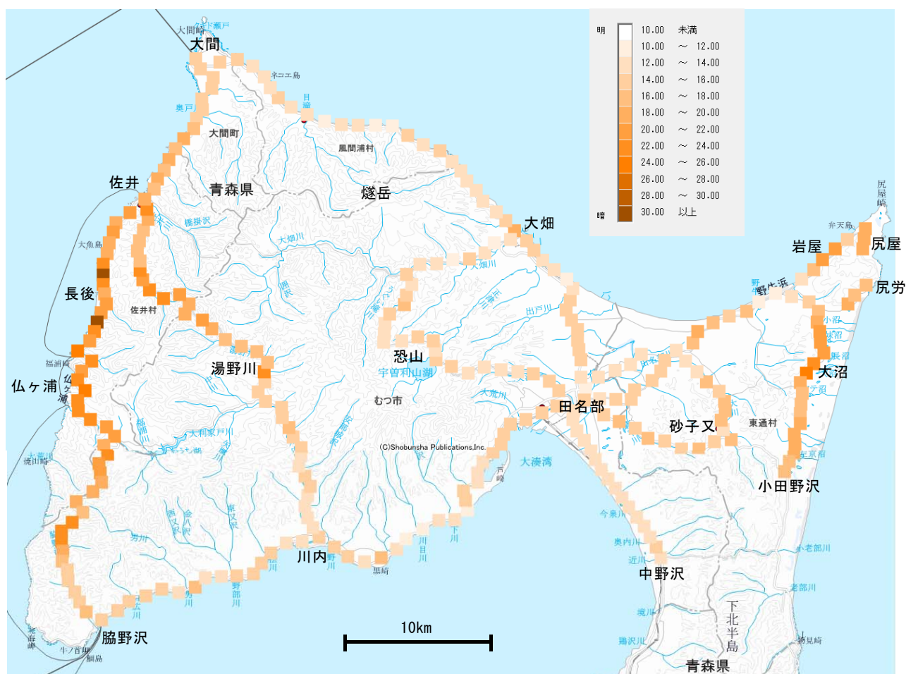
図 6 サーベイカーによる走行測定結果
