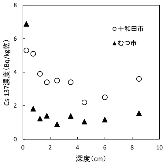
図4 土壌中 Cs-137 の深度分布状況
