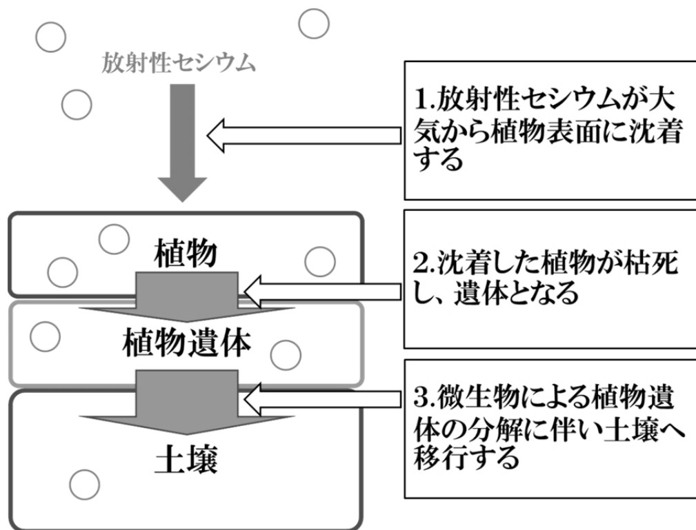
図4 採取地点における放射性セシウムの移行挙動概念図
