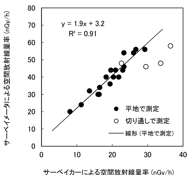
図 7 サーベーカーとサーベイメータによる定点測定比較結果
