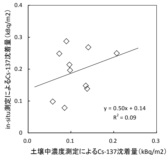
図5 土壌中濃度測定と in-situ 測定による Cs-137 沈着量の関係 (ND のデータは除外)
